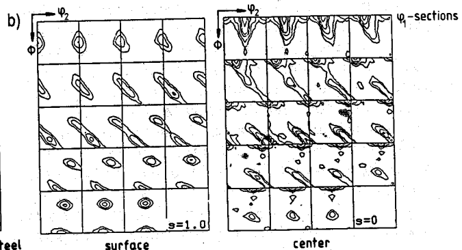
Bild 8b. Warmwalztextur von Oberfläche und Mitte eines Fe16%Cr-Stahls
